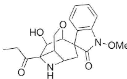
gelsemoxonine
